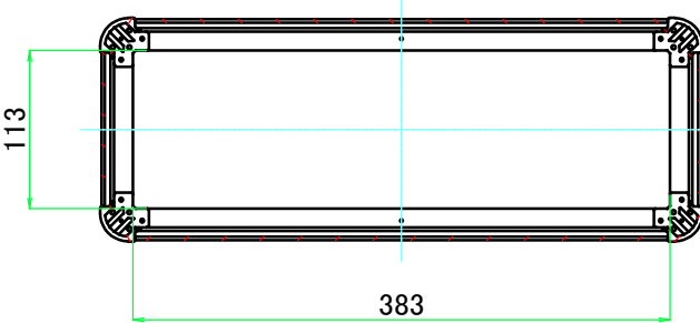
C-C ( 1 : 6 )
